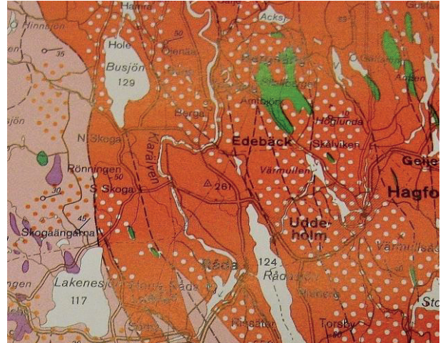
Berggrunden runt Edebäck. Gnejs i väster, granit i öster. Gräns mellan gnejsen och graniten utgörs av Protoginzonens västgräns
